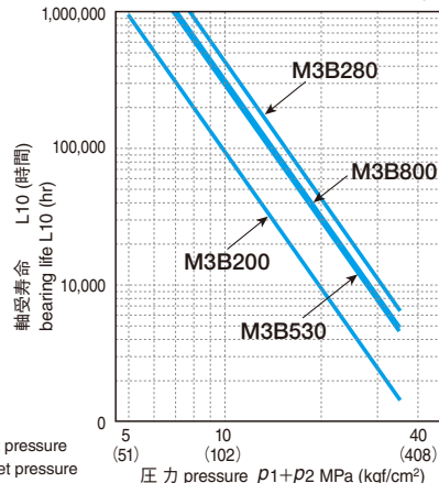
◆フロント軸受寿命 / Front bearing life
