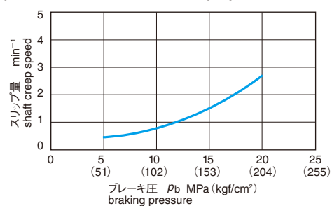
◆保持特性 / Shaft creep speed
