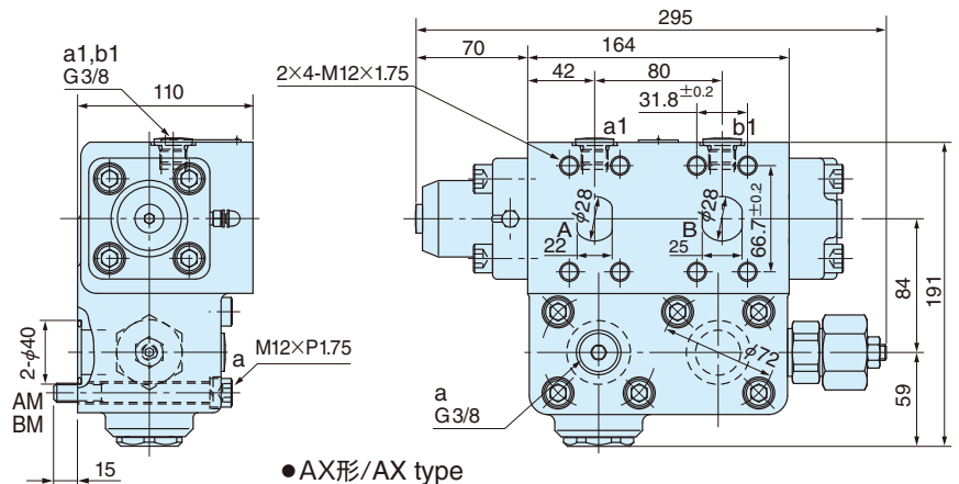
●AX形/AX type
