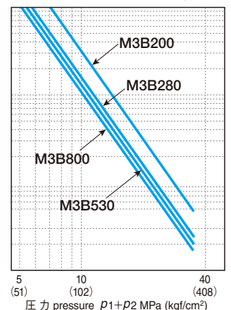
◆リア軸受寿命 / Rear bearing life
