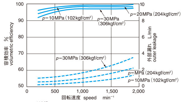
◆容積効率・外部リーク / Volumetric efficiency
