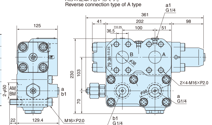
●AX形/AX type
